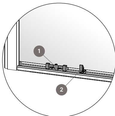
1. Dispositivo regolazione altezza vetro 2. Ferma vetro
