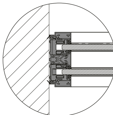
Dettaglio profilo di partenza
